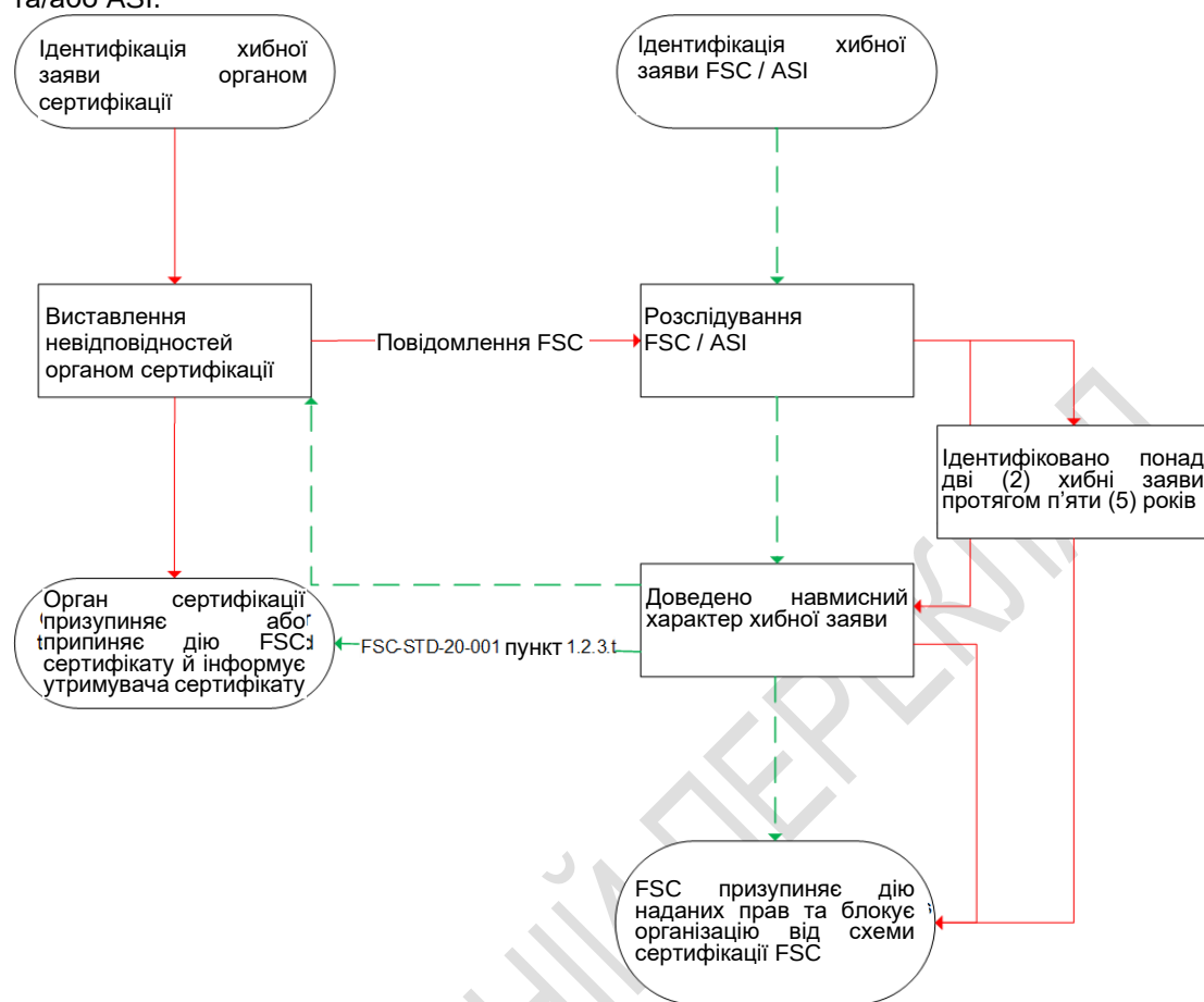
Рис. 2. Блок-схема обробки випадків ідентифікації хибних заяв органами сертифікації та/або ASI.
